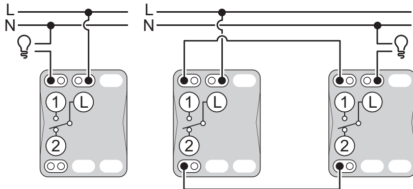
Dvopoložajni sklop
