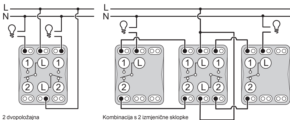
2 dvopoložajna sklopa
