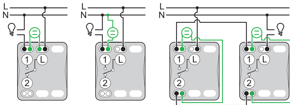
Dvopoložajni sklop s lokatorskom lampom
